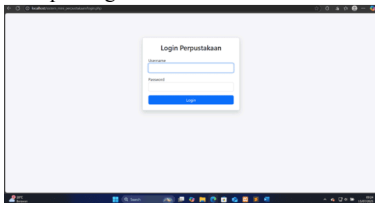
Gambar 2. Halaman Login
